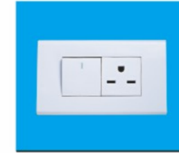
ZH 203 ZH 203 3way 10A 125V 6A 250V 15A 125V/250V
