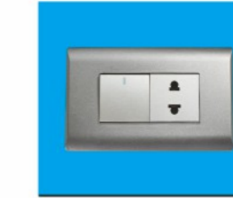
ZKG 108 ZKG 108 3way 10A 125V 6A 250V 16A 127V/250V
